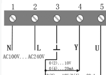
Volt0(0)...10V input resistance≥200KΩ Uurrent0(4)...20mA input resistance=500Ω
